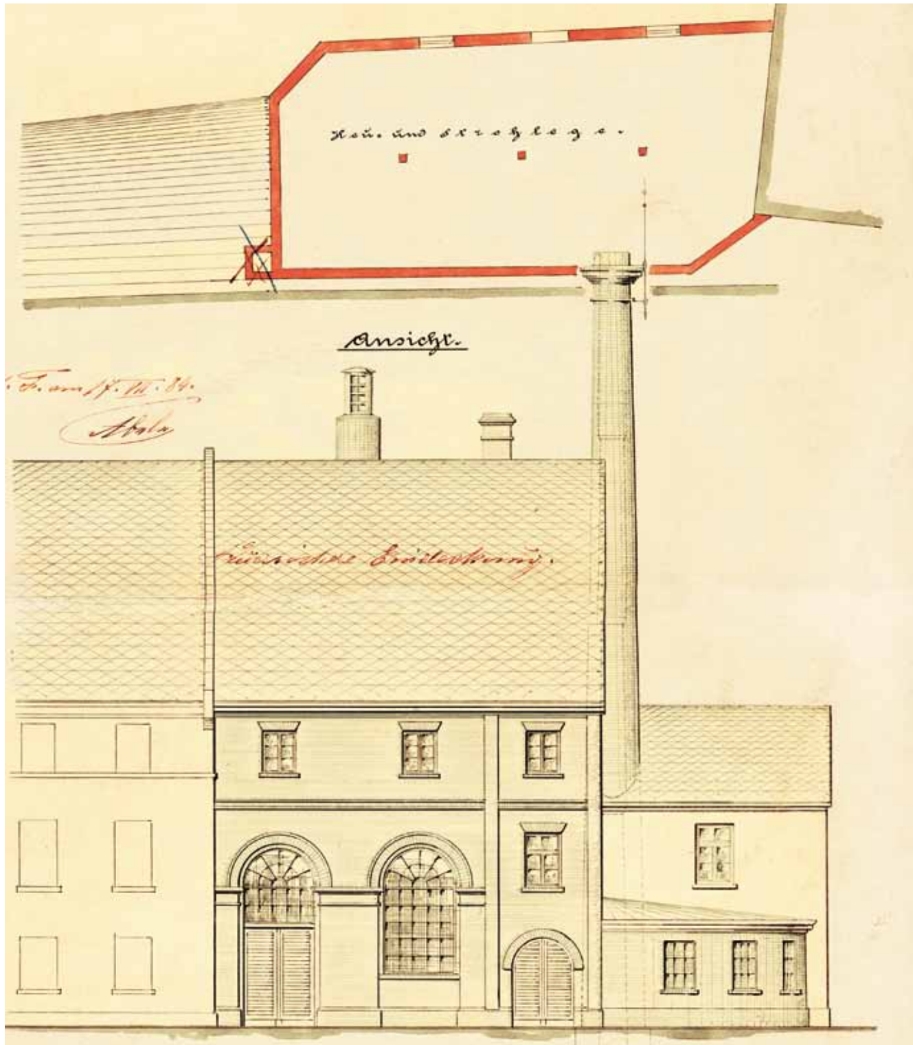
01 Fassaden-Aufriss zum Neubau des Sudhauses in der Urban-Brauerei, Heinrich Lang, 1880 (Stadtarchiv Freising, Historische Bauakten)
